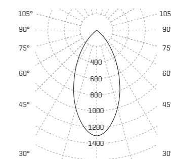
Abstrahlwinkel 55°
