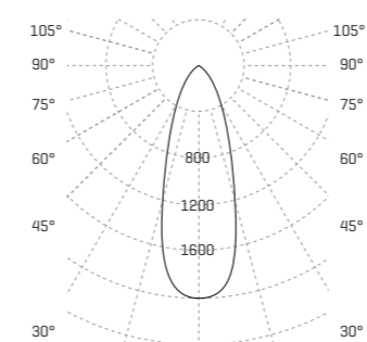
Abstrahlwinkel 25°
