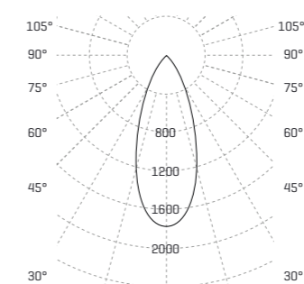
Abstrahlwinkel 35°
